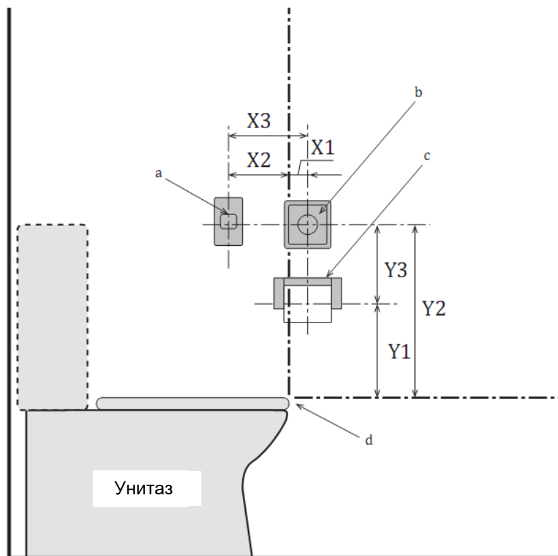
Рисунок 1 – Схема расположения кнопки смыва, кнопки вызова и держателя бумаги
